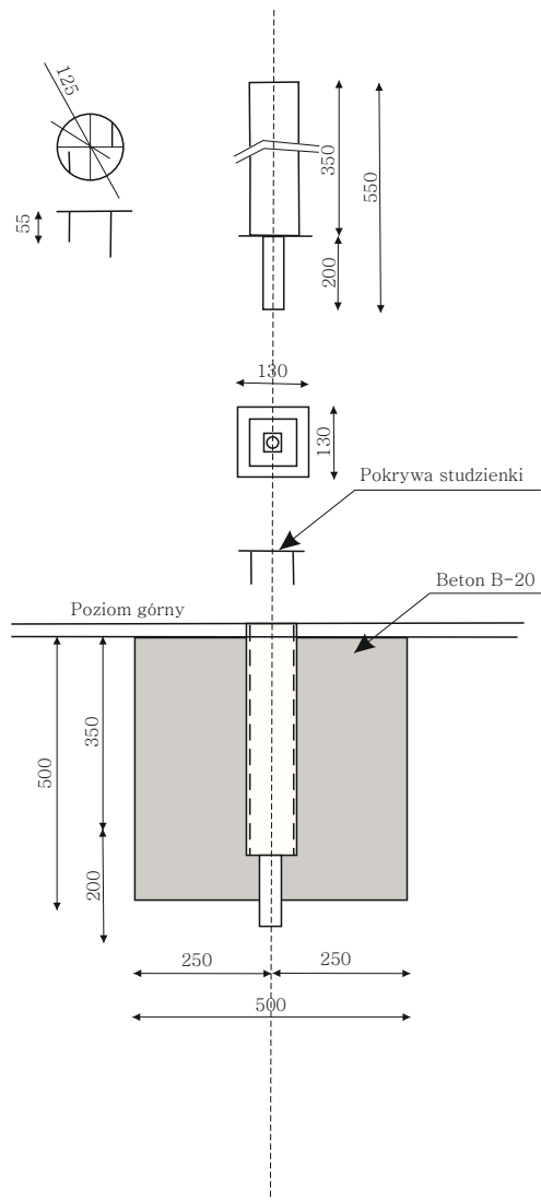
Studzienka z fundamentem maszt do piłki ręcznej
