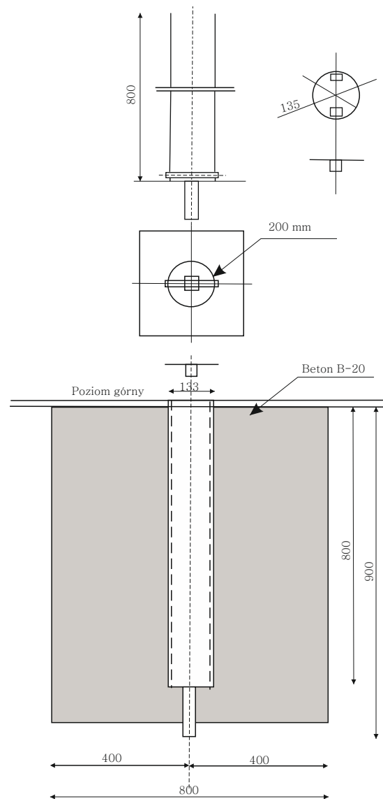
Studzienka z fundamentem maszt do koszykówki
