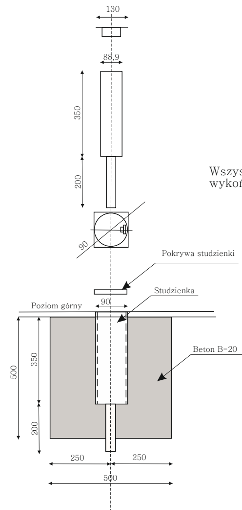
Studzienka z fundamentem maszt do siatkówki – tenis
