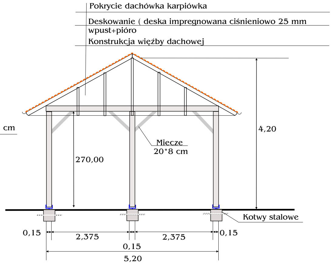
Przekrój pionowy
