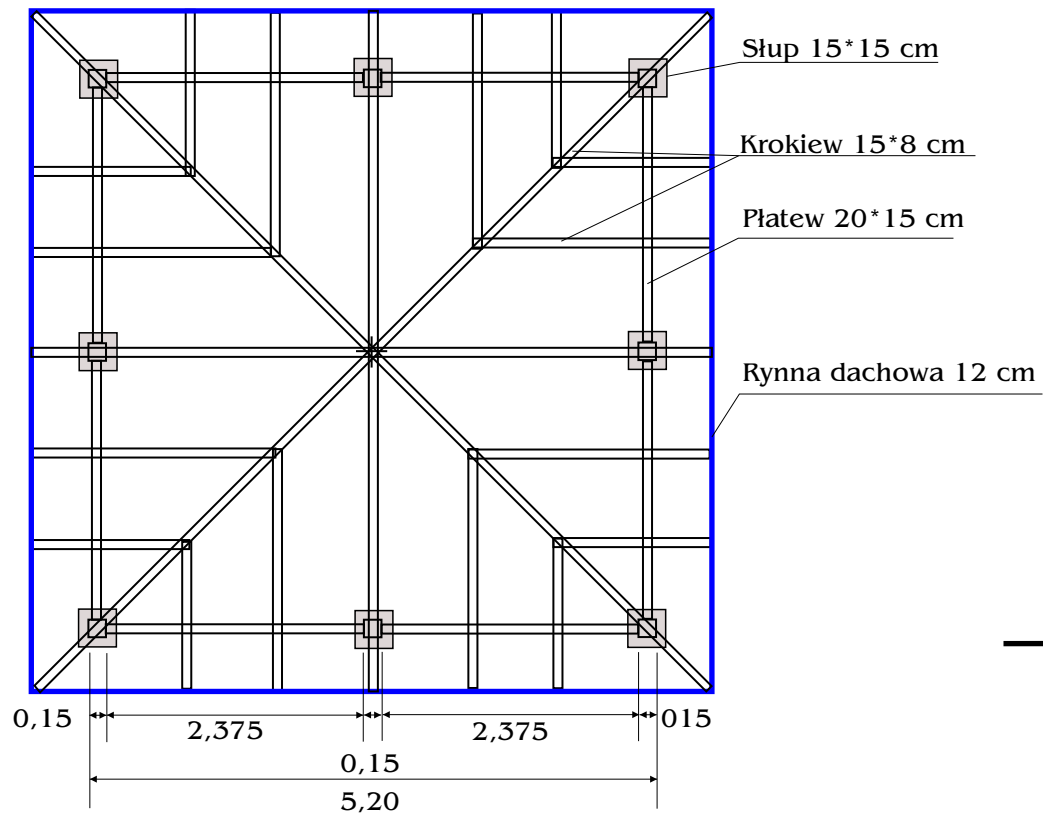
Rzut poziomy
