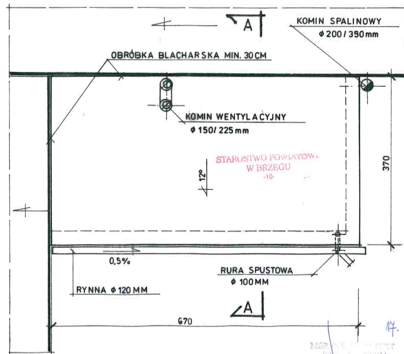
rzut dachu skala 1:50
