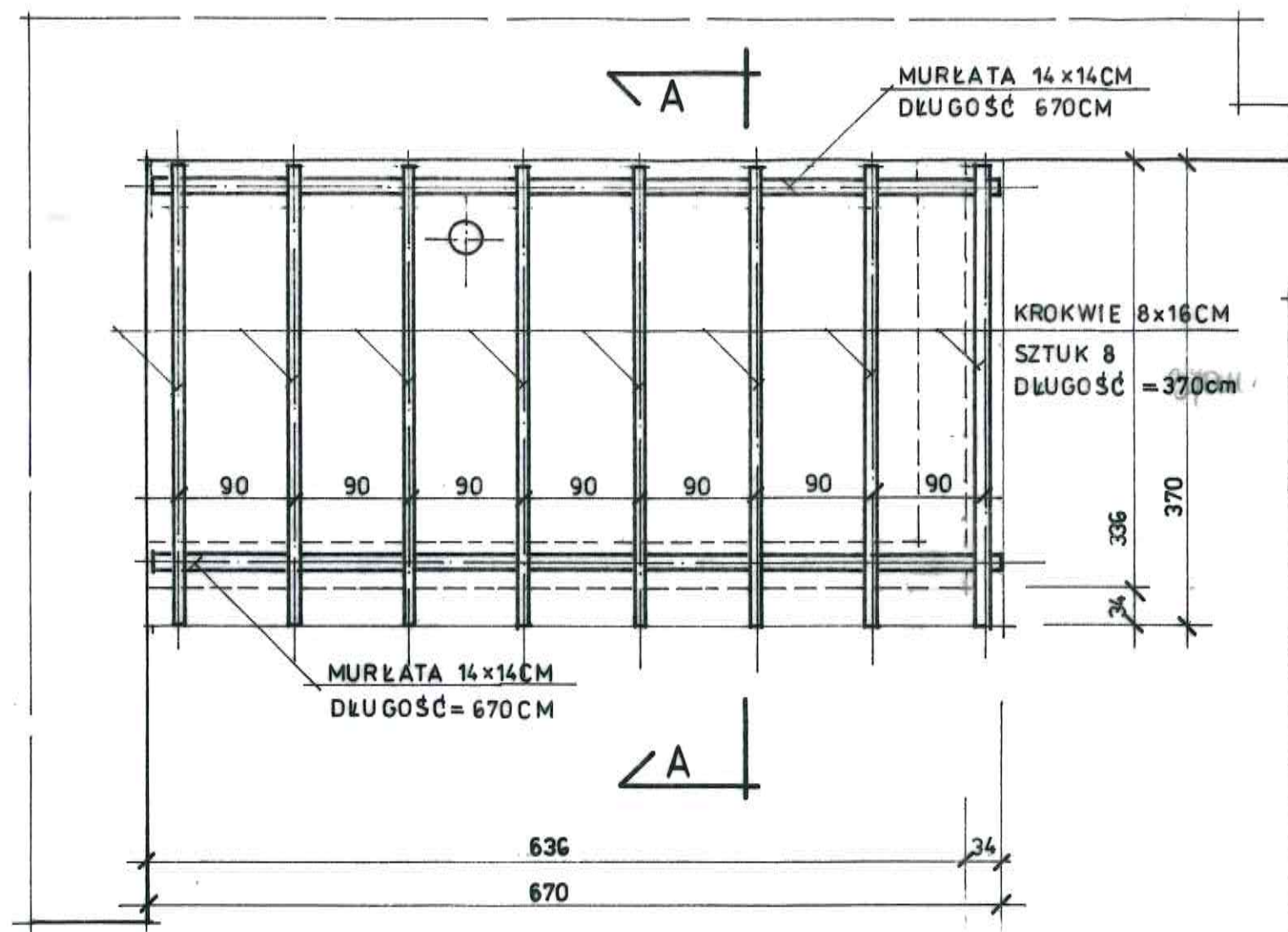
rzut więźby dachowej skala 1:50
