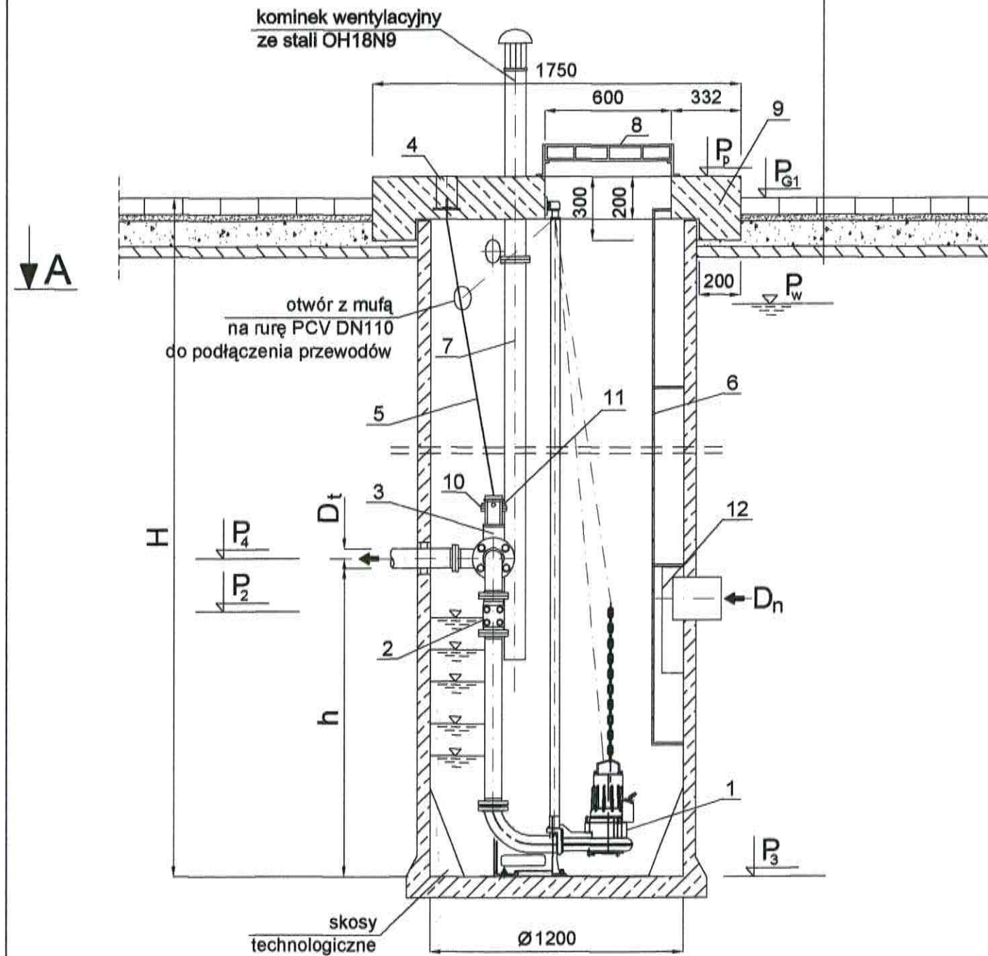
PRZEKRÓJ PIONOWY skala 1:25
